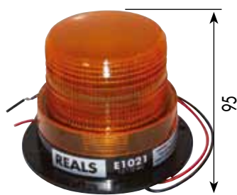
Feu à éclats Flashing strobe beacon Entraxe de fixation Fixing points : 100 12-110 V E1021 - 554947
